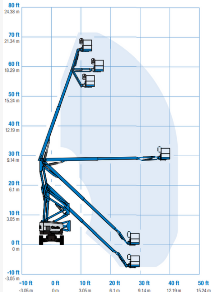
Diagrama de trabajo Z-62/40
